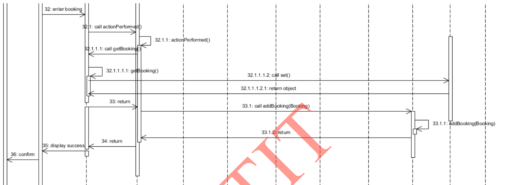
Hình 8.24: Sơ đồ tuần tự cho chức năng đặt phòng, thiết kế theo mô hình MVC cải tiến
