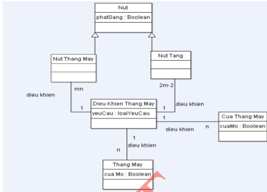
Hình 8.9 Vòng lặp thứ ba của biểu đồ lớp
