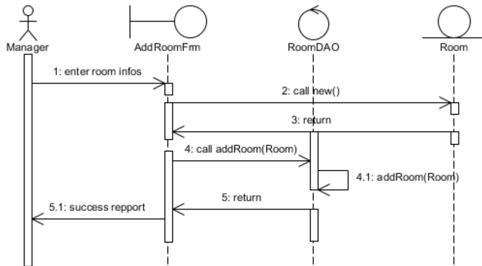
Hình 8.16: Sơ đồ tuần tự cho chức năng thêm thông tin phòng, thiết kế dùng DAO và thực thể tuần
